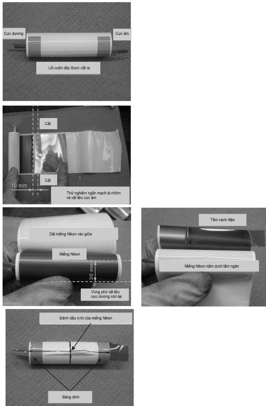
Hình A.4 - Tháo tế bào hình trụ
